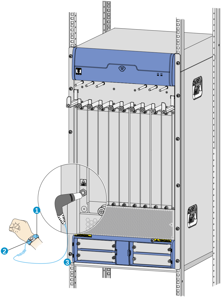
图1-1 佩带防静电腕带示意图
