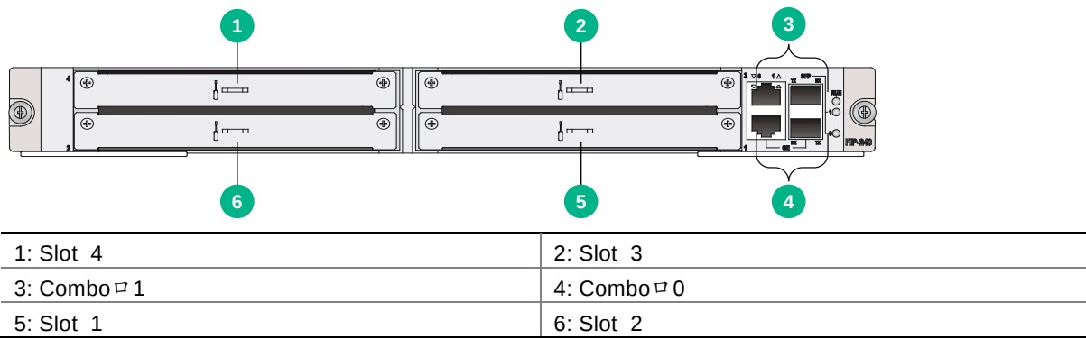
图A-11 FIP-240 正视图
