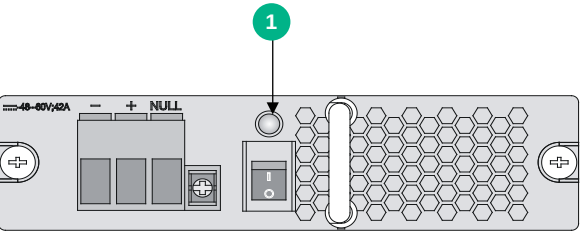
图B-12 PSR1200-D 直流电源模块指示灯
