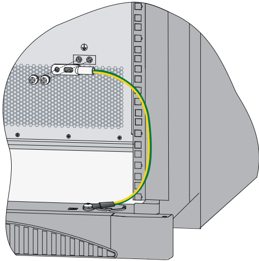
图2-7 连接保护地线到接地排
