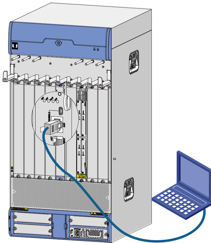
图4-1 连接 Console 口电缆
