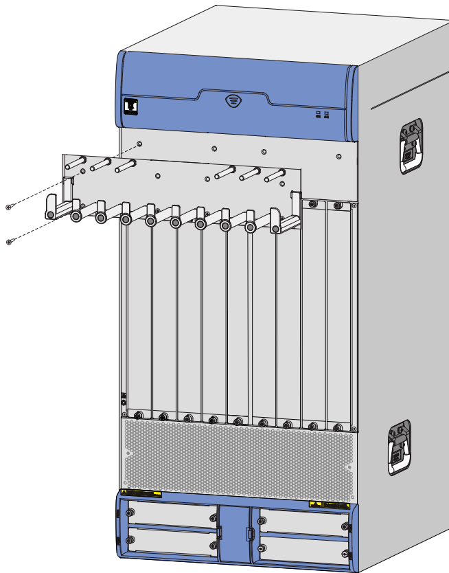
图2-4 安装 R7900-16 的走线架
