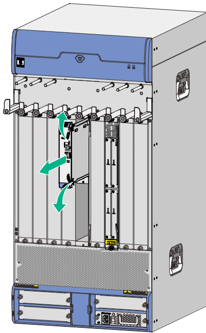
图6-2 将主控板拉出主控板插槽
