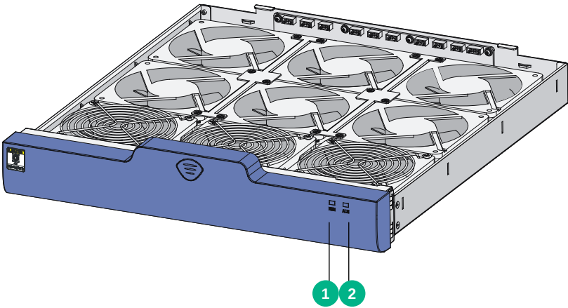
图B-13 R7900-16 的风扇框结构图
