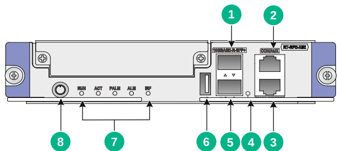
图A-10 主控板RPE-X5E 正视图
