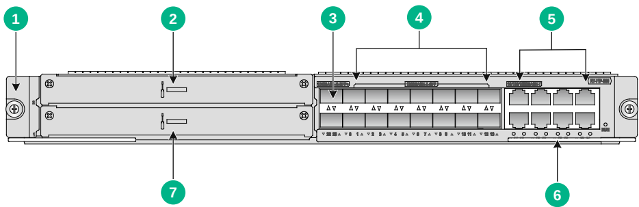
图A-15 FIP-380 正视图
