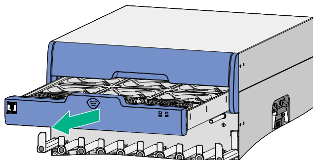
图6-6 将风扇框拉出风扇框插槽
