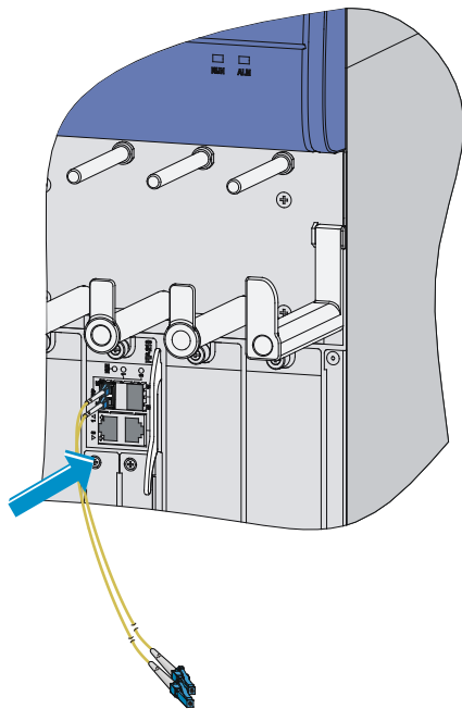
图3-9 LC 光纤连接器连接光模块
