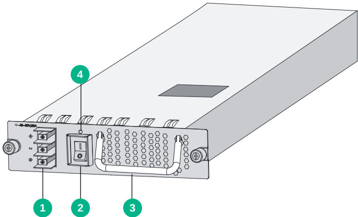
图A-5 PSR650-D 直流电源模块外观
