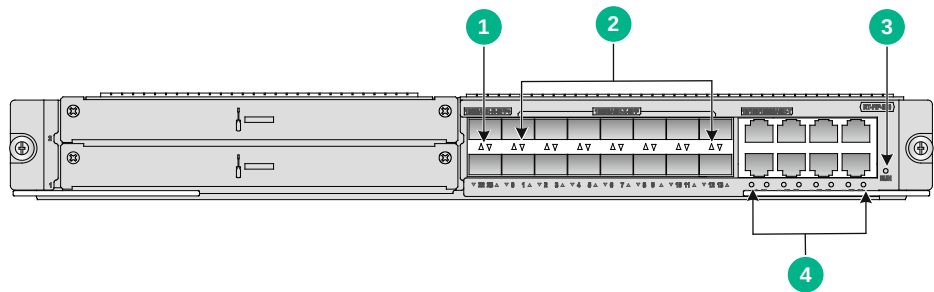
图B-8 FIP-380 指示灯
