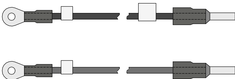
图2-15 直流电源线示意图（适用于 PSR650-D 直流电源模块）
