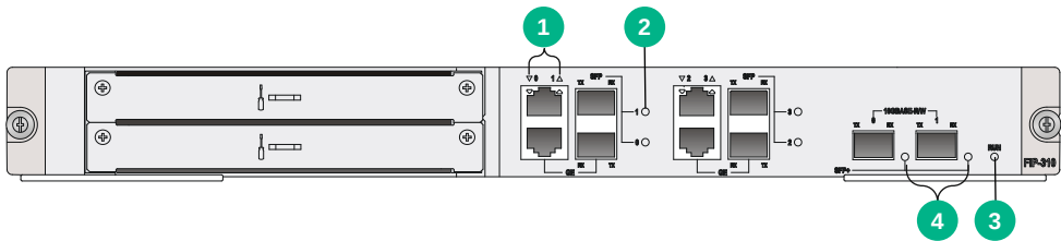
图B-7 FIP-310 指示灯
