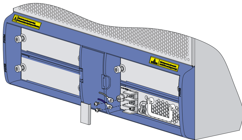
图2-16 连接直流电源线
