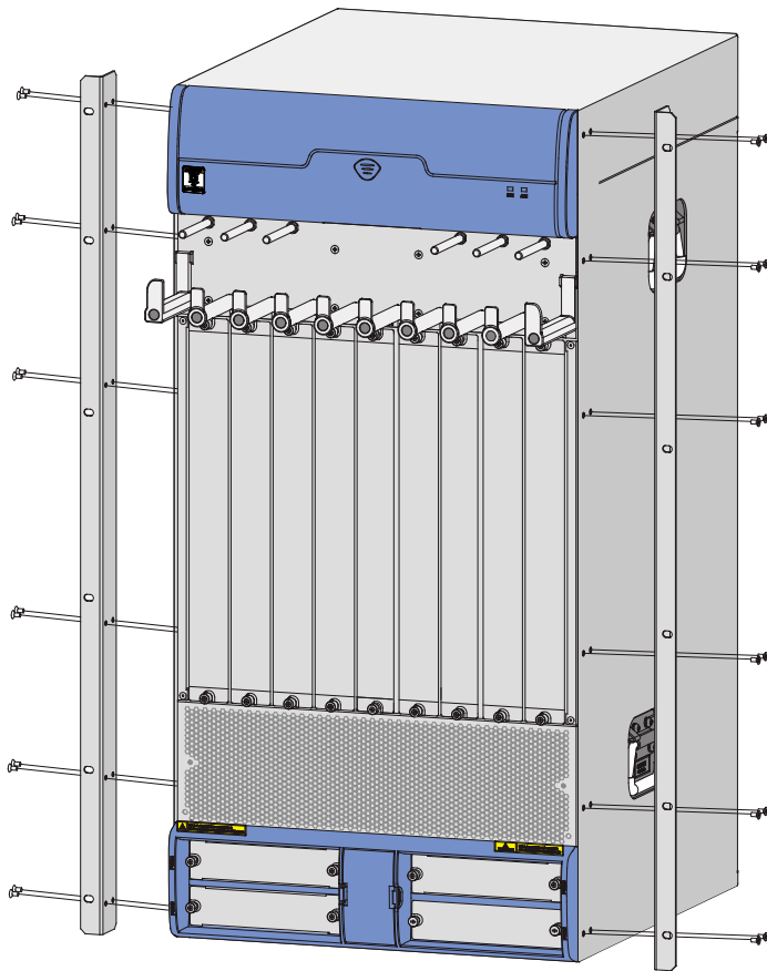
图2-5 安装挂耳到设备的两侧
