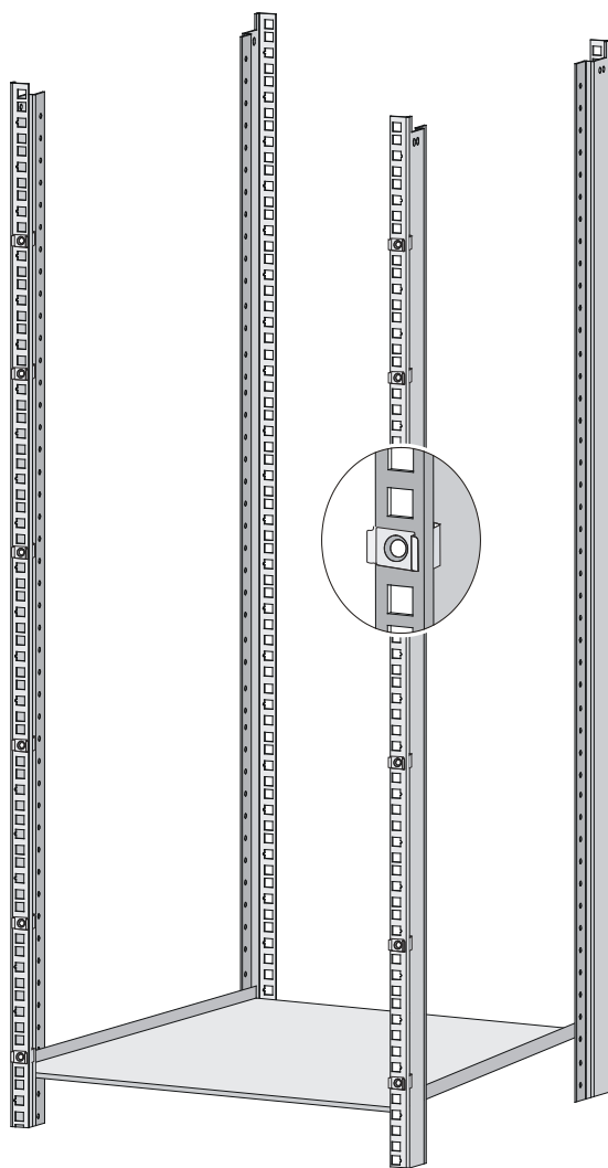
图2-3 安装浮动螺母
