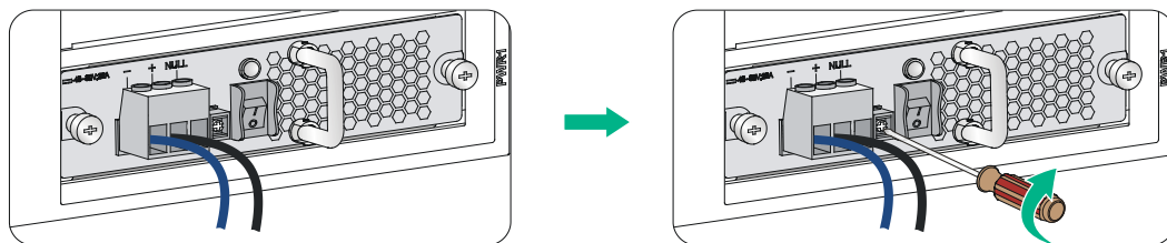
图2-19 将电源连接器安装到电源模块
