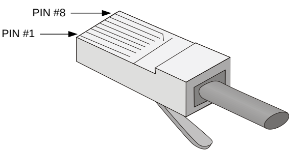
图3-3 RJ-45 连接器引脚序号示意图
