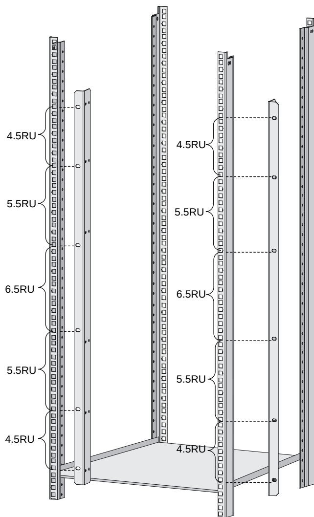
图2-2 标记浮动螺母的安装位置
