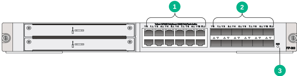
图B-6 FIP-300 指示灯
