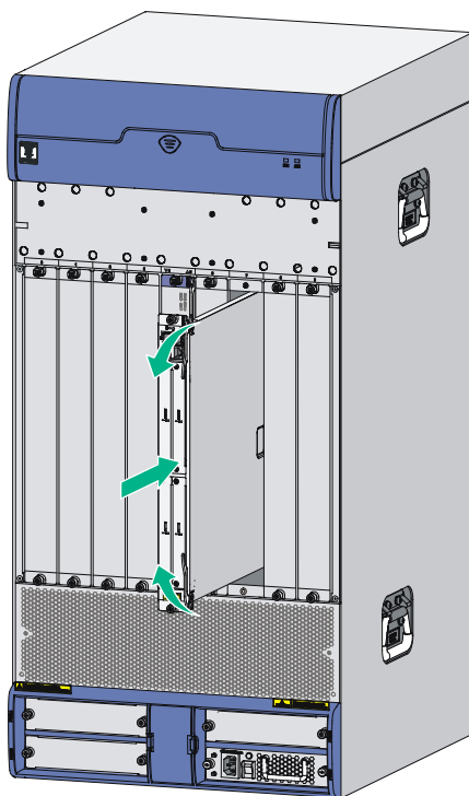
图2-10 将 FIP 板插入业务板插槽
