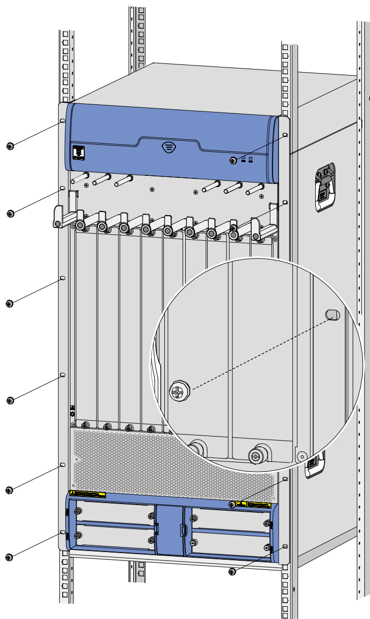
图2-6 固定设备到机柜
