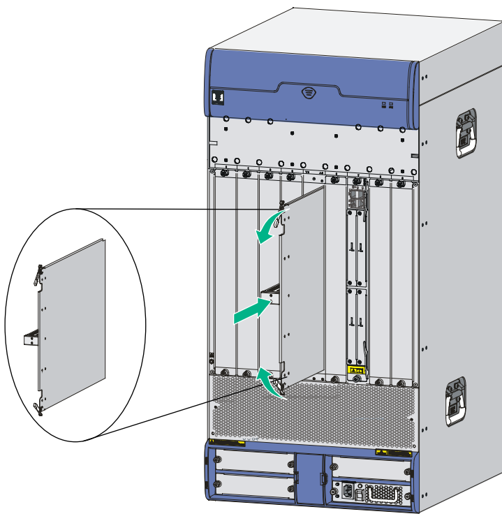
图2-8 安装托板
