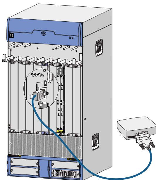
图3-2 AUX 口线缆连接示意图
