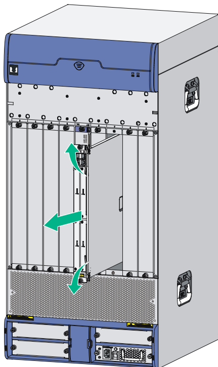
图6-3 将 FIP 板拉出业务板插槽
