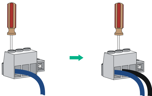
图2-18 将直流电源线安装到电源连接器
