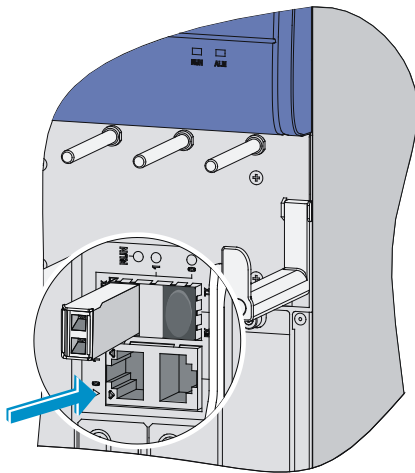
图3-8 插入光模块
