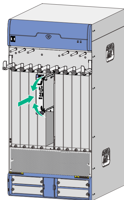
图2-9 将主控板插入主控板插槽
