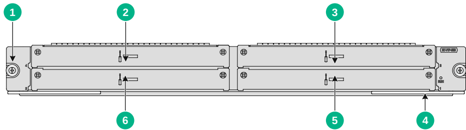
图A-12 FIP-260 正视图
