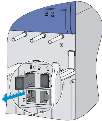
图3-7 取下防尘盖
