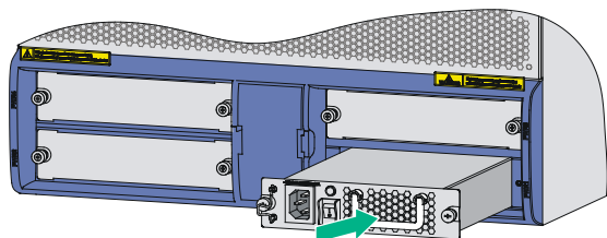
图2-13 将电源模块插入电源插槽
