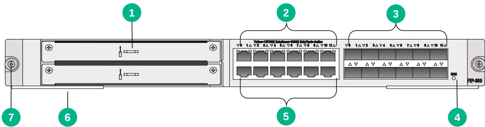
图A-13 FIP-300 正视图
