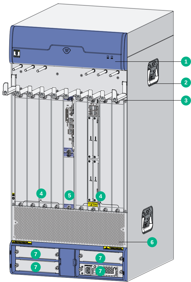
图A-1 R7900-16 前视图（配置 RPE-X3/RPE-X5/RPE-X5E 主控板）
