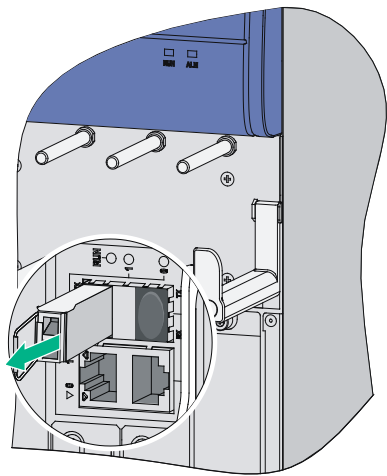
图6-5 拆卸可插拔接口模块示意图
