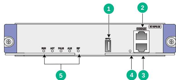
图A-9 主控板 RPE-X5 正视图
