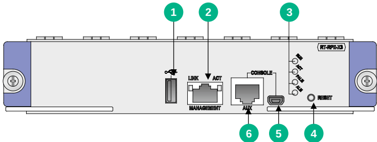
图A-8 主控板 RPE-X3 正视图
