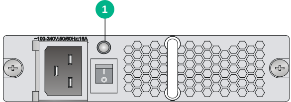
图B-10 PSR1200-A 交流电源模块指示灯
