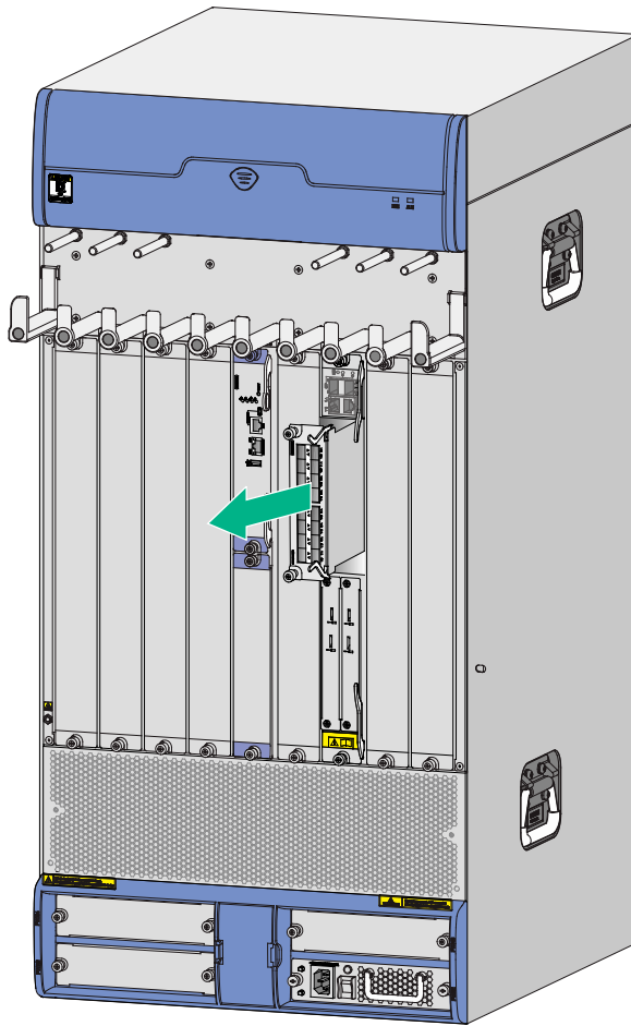
图6-4 将 MIM 从 MIM 插槽中拉出
