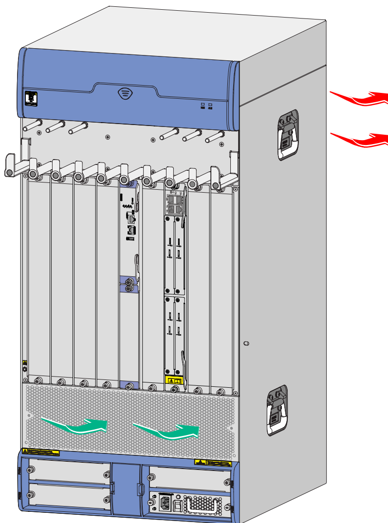
图1-2 设备的散热方式
