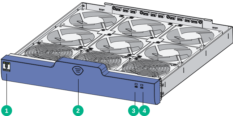
图A-7 风扇框结构图
