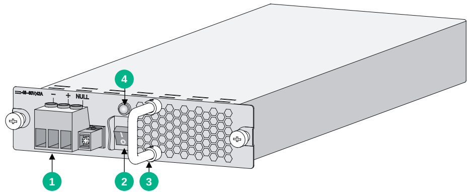
图A-6 PSR1200-D 直流电源模块的外观
