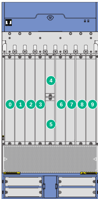
图C-1 R7900-16 的槽位排列顺序
