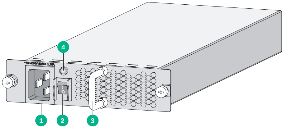
图A-4 PSR1200-A 交流电源模块外观
