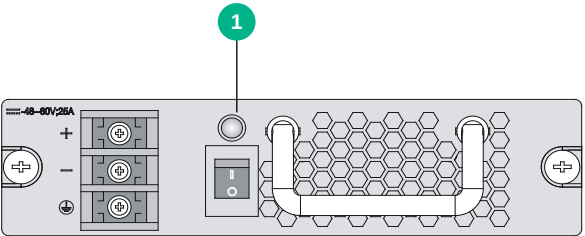
图B-11 PSR650-D 直流电源模块指示灯
