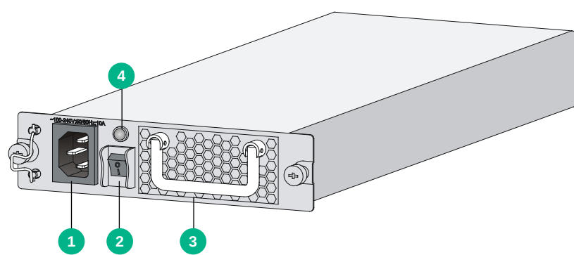
图A-3 PSR650-A 交流电源模块外观
