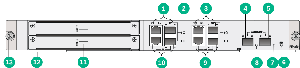
图A-14 FIP-310 正视图
